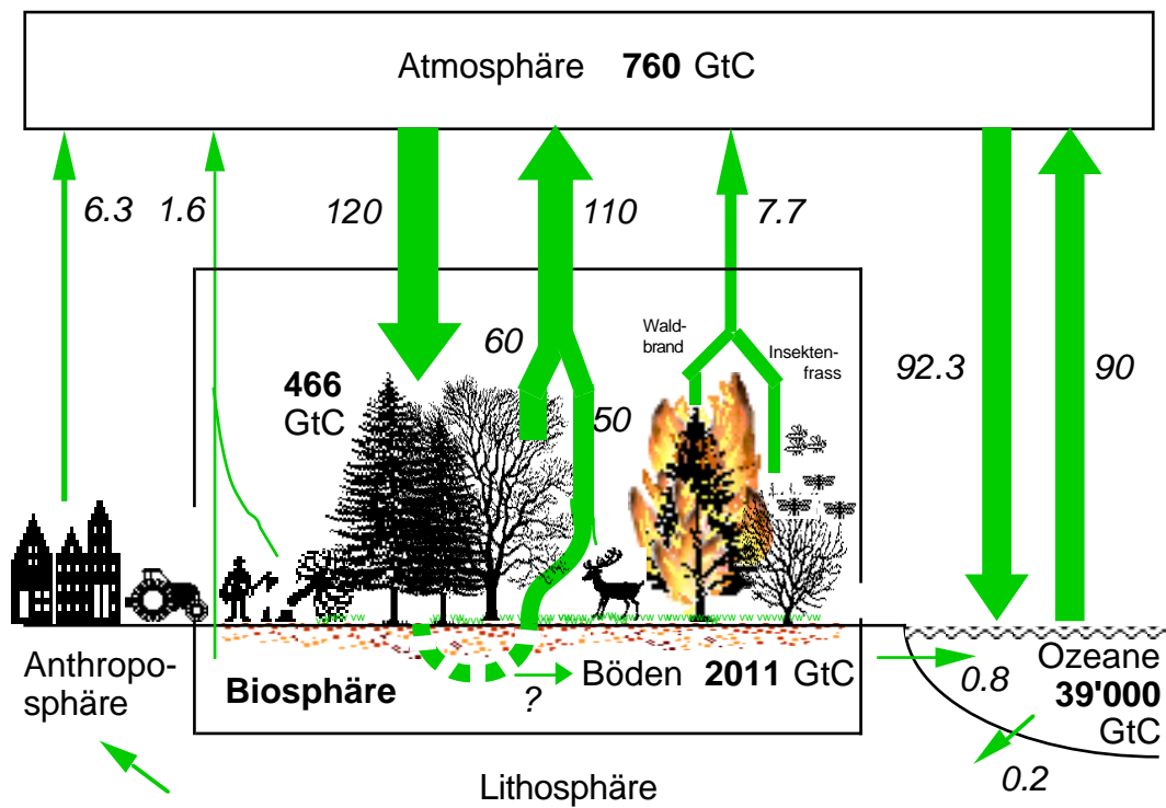
Der globale Kohlenstoffkreislauf. Die fett gedruckten Zahlen stehen für Kohlenstoffvorräte, die kursiven für jährliche Kohlenstoffflüsse in Gigatonnen (GtC). (Grafik Fischlin / Daten IPCC)
