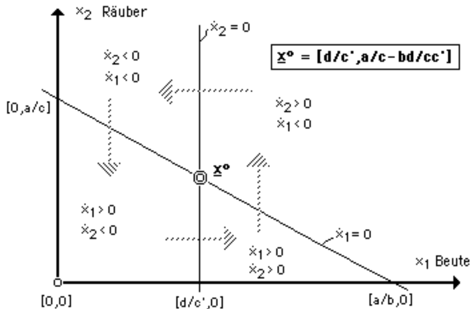
Fig. 2: Gleichgewichtslagen im Zustandsraum eines nichtlinearen Differentialgleichungssystemes zweiter Ordnung (Lotka-Volterra Räuber-Beute Modell).
