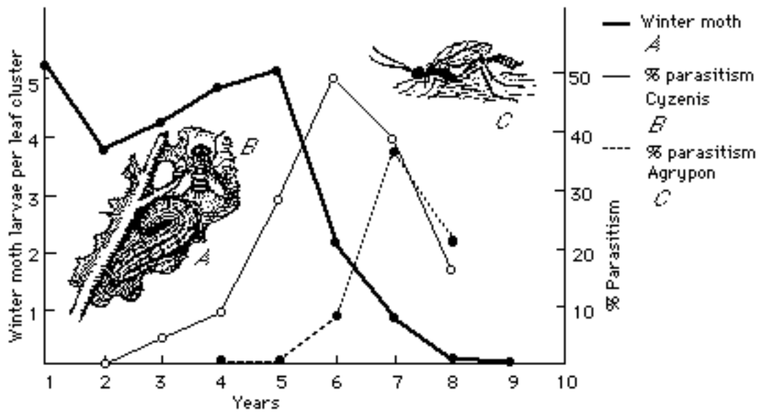
Fig. 3: Verhalten der Schädlings- und Parasitoidenpopulationen des Frostspanners Operophtera brumata , der in den Obstanlagen von Nova Scotia, Kanada, zu Beginn dieses Jahrhunderts Schaden verursachte, und dessen Parasitoiden Cyzenis albicans . Seit der Einführung des Parasitoiden, erster Nachweis 1954, ist die Schädlingspopulation auf den angezeigten, niedrigen Werten verblieben (nach Varley et al., 1973).
